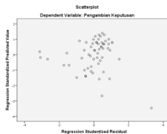
Gambar 2. Hasil Uji Normalitas
