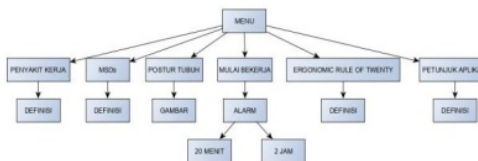
Gambar 4. Hierarki Menu pada Aplikasi Kerja Sehat
