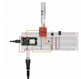
Gambar 2. Desain Rangkaian IoT Loadcell
