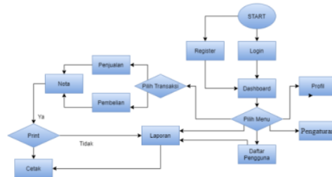
Gambar 7. Flowchart Aplikasi
