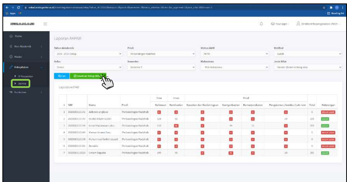
Gambar 2.37 Contoh AKPAM
