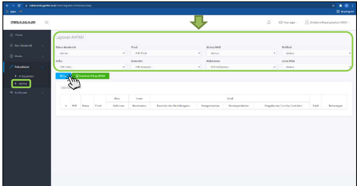
Gambar 2.36 AKPAM
