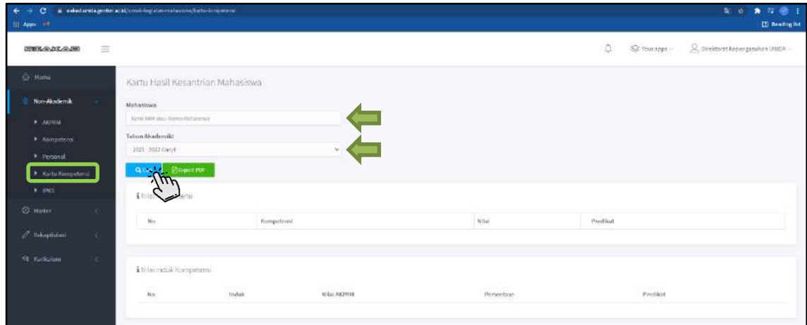
Gambar 2.15 Kartu Kompetensi
