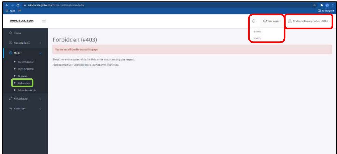
Gambar 2.31 Mahasiswa
