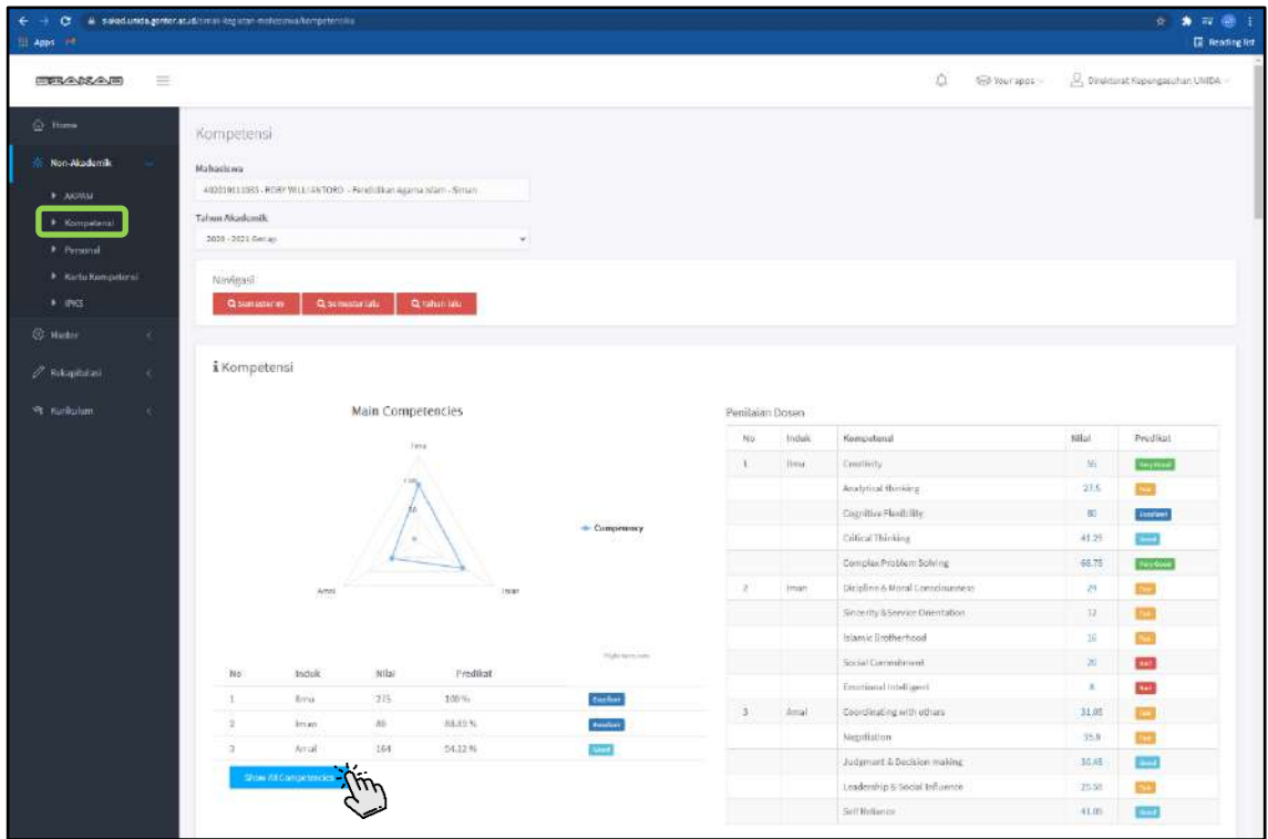
Gambar 2.11 Contoh Kompetensi
