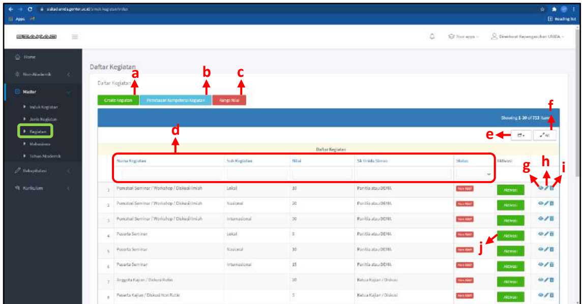
Gambar 2.27 Kegiatan
