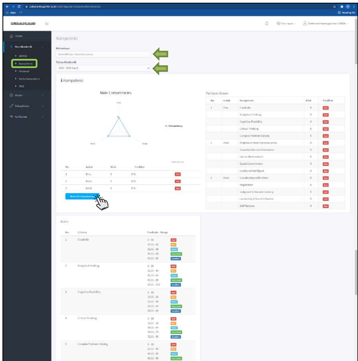
Gambar 2.10 Kompetensi
