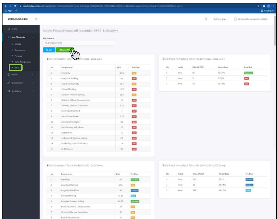
Gambar 2.19 Contoh IPKS
