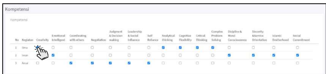
Gambar 2.23 Pemetaan Kompetensi
