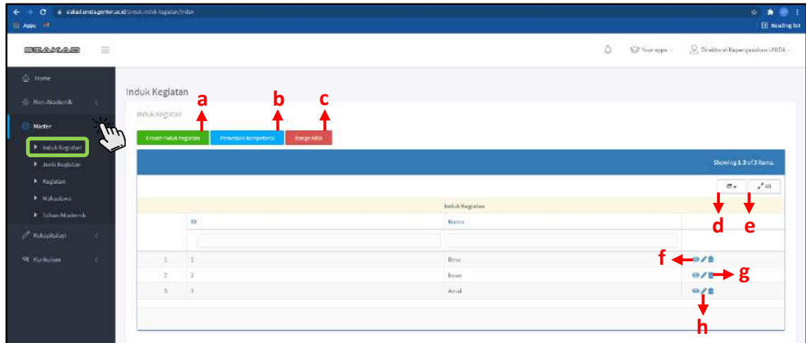
Gambar 2.21 Induk Kegiatan
