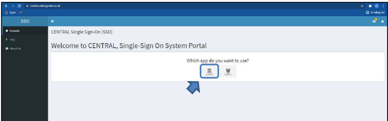
Gambar 2.1 SIAKAD
