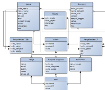
Gambar 3. ERD sistem pakar
