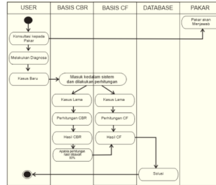
Gambar 2. Activity diagram sistem Pakar Penyakit Bawang Merah
