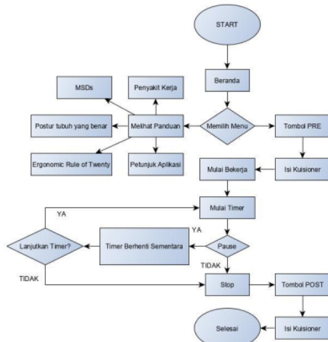
Gambar 3. Flowchart Alur Proses Aplikasi
